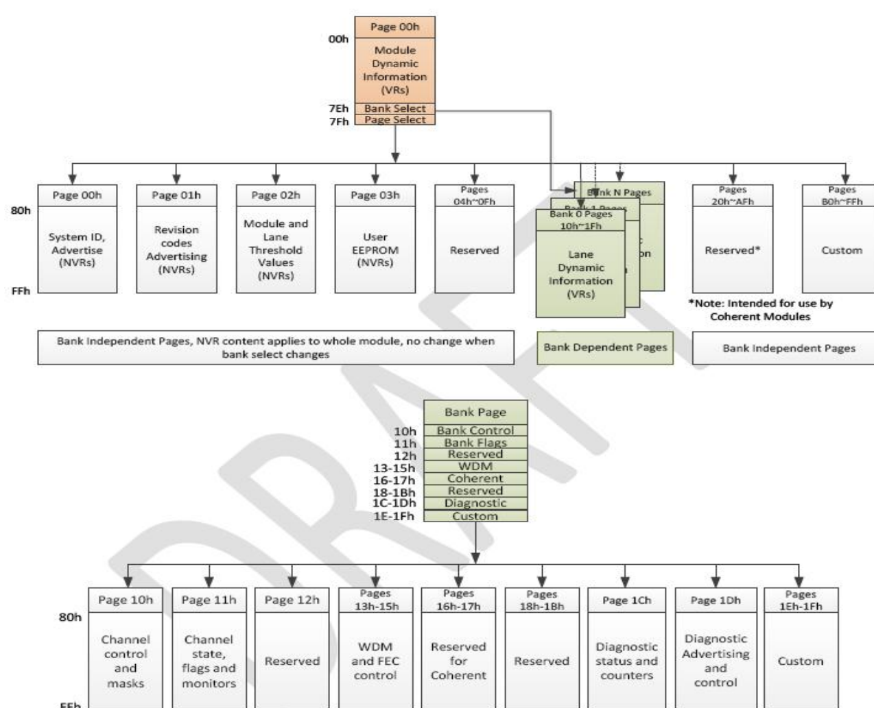
Figure6. QSFP-DD Memory Map
