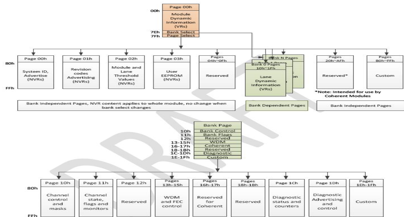
Figure6. QSFP DD Memory Map
