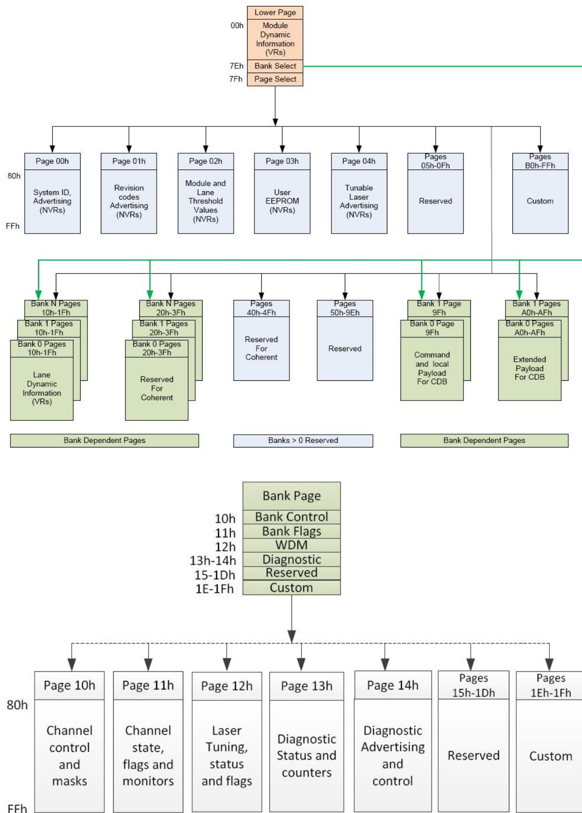
Figure4. Memory Map
