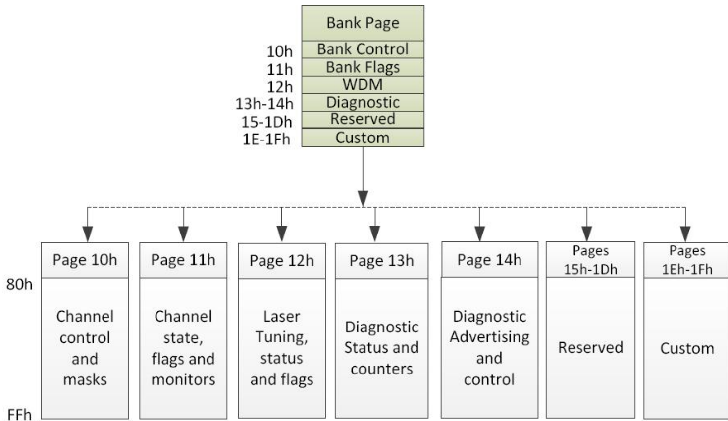
Figure4. QSFP112 Memory Map
