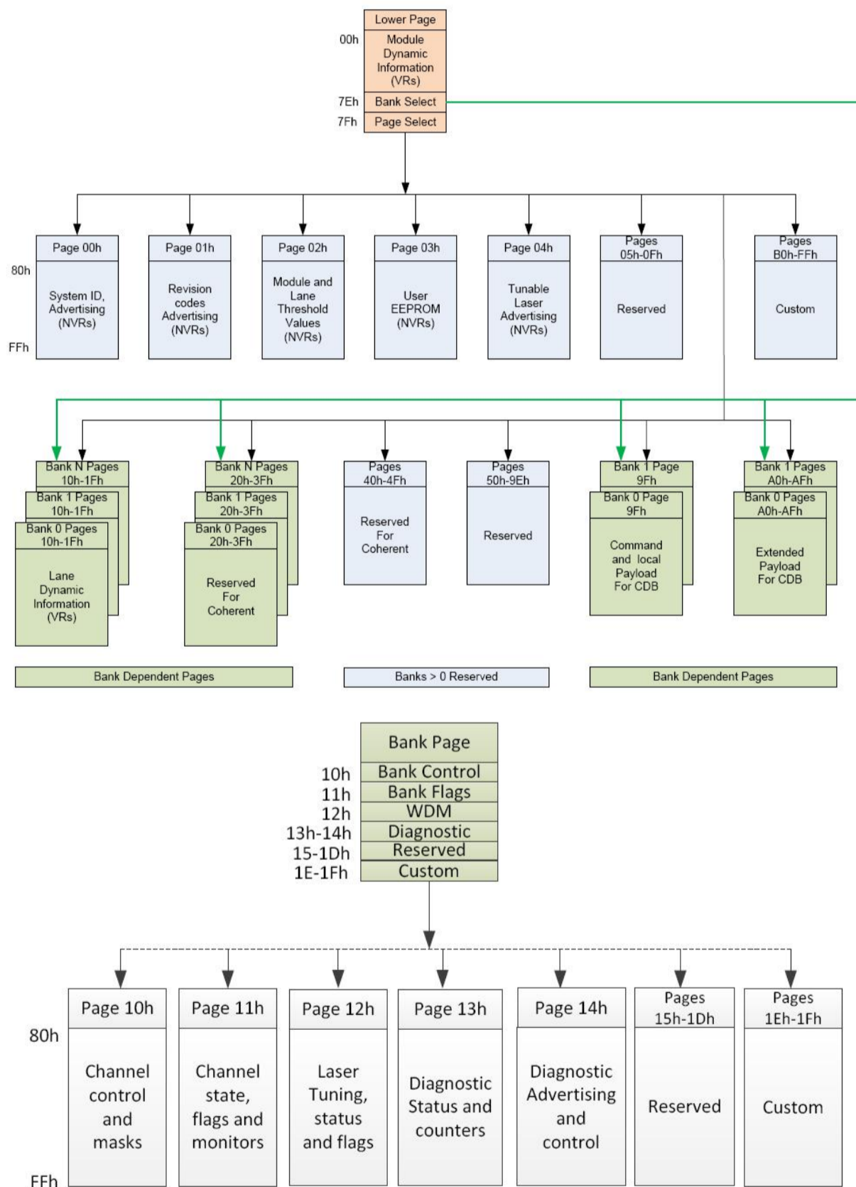
Figure5. QSFP DD Memory Map
