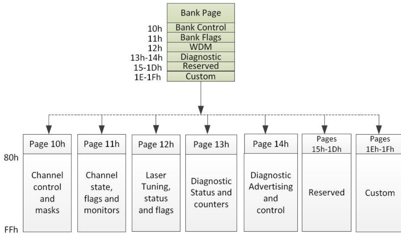
Figure4. QSFP DD Memory Map
