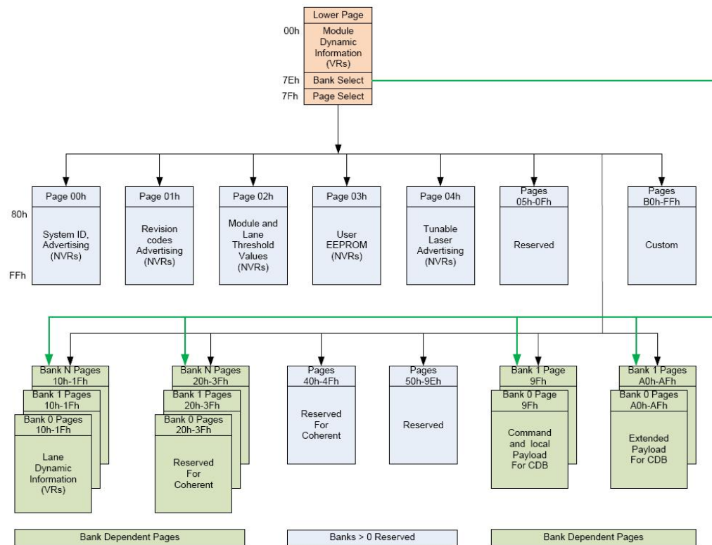
Figure4. QSFP DD Memory Map
