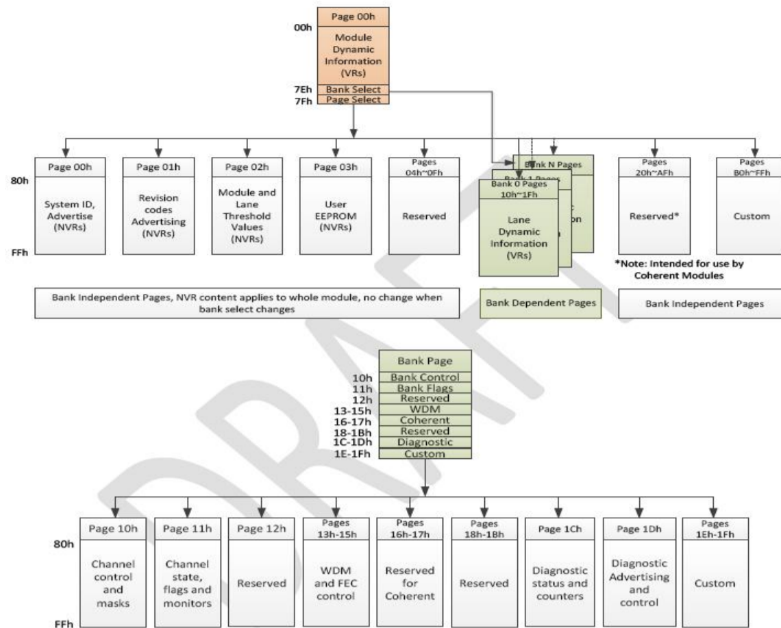
Figure4. QSFP DD Memory Map
