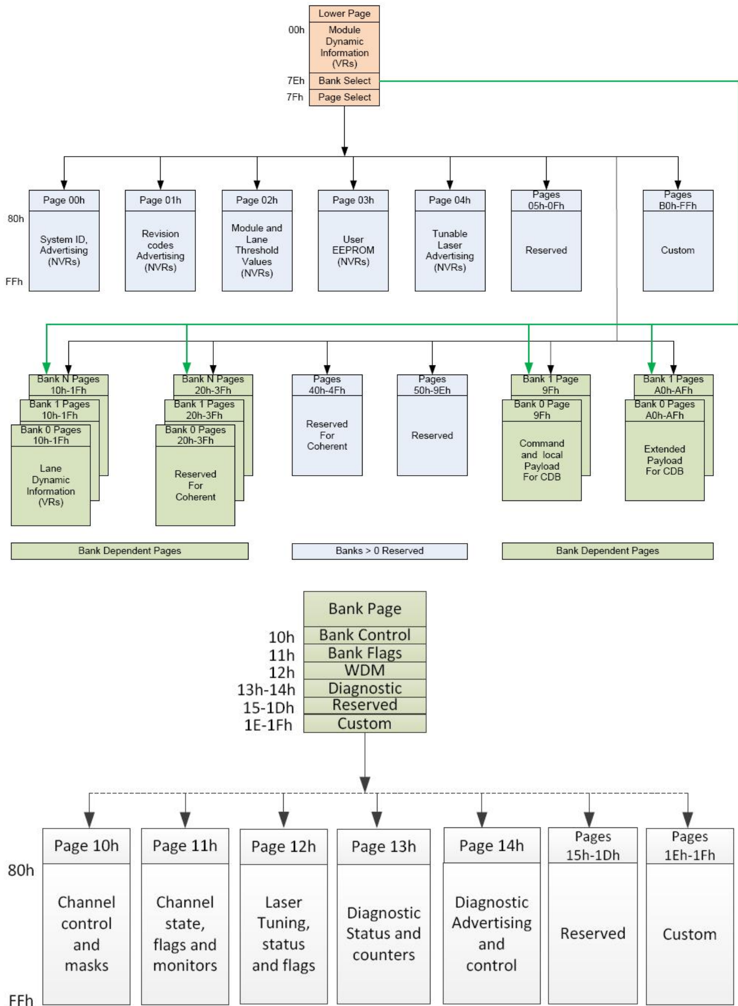
Figure5. QSFP DD Memory Map
