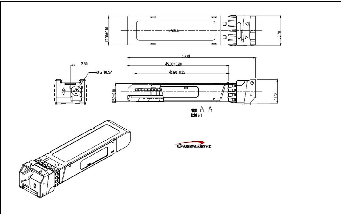
1.1.1.1. Figure4. Key Mechanical Dimensions
